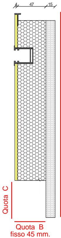
Sezione SPALLA TERMICA RIFINITA Spessore 6 cm.
