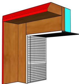
Telaio in OSB con Rete e XPS
