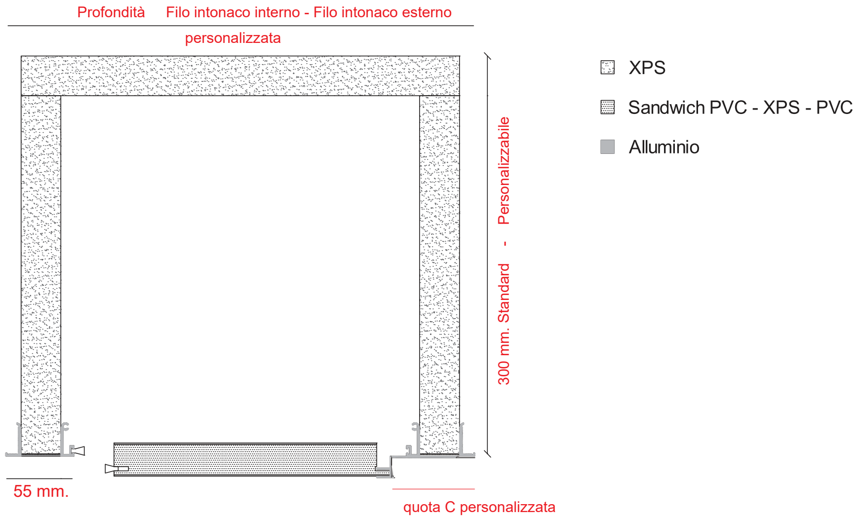
Sezione CASSONETTO ISPEZIONE A TAMPONE muro foro passante Infisso filo intonaco interno
