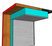
Spalla Rifinita per Infisso e Persiana
